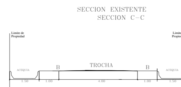
TROCHA CARROZABLE LATERAL AL PREDIO ESC. 1/200
