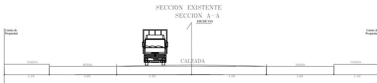
CARRETERA CAÑETE-LUNAHUANA-ZUNIGA ESC. 1/200
