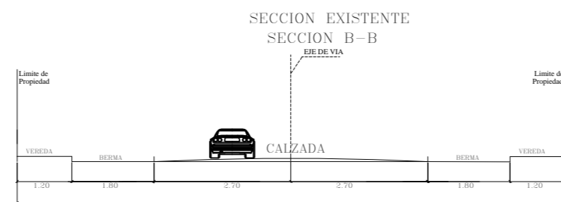
CALLE DE ACCESO HACIA EL TERRENO ESC. 1/200
